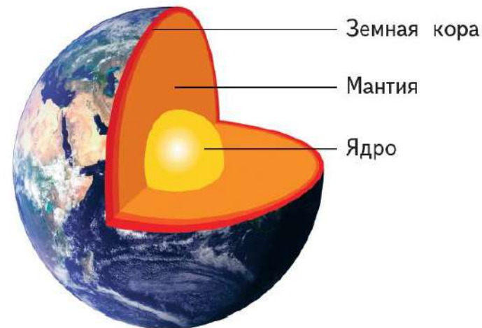
Внутреннее строение Земли
